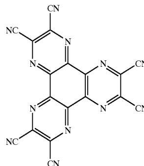
Hexanitride hexaazatriphenylene
