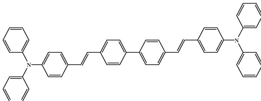
DSA amine
